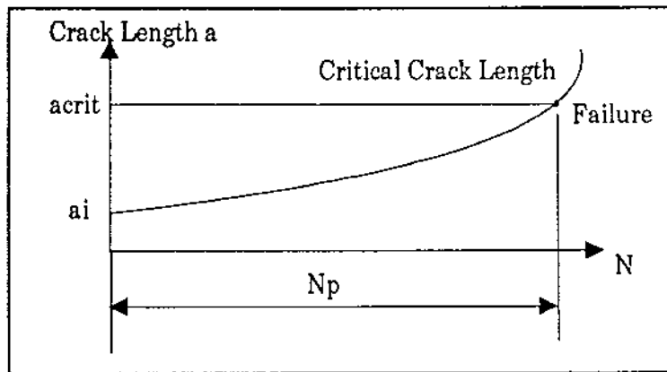
Fig. 4.5 Fatigue Life N_p
